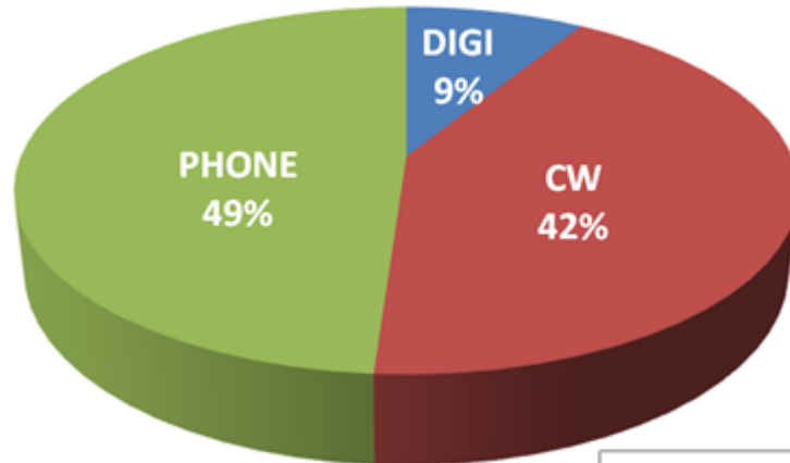
FD 2015: QSO(%) Per Mode
