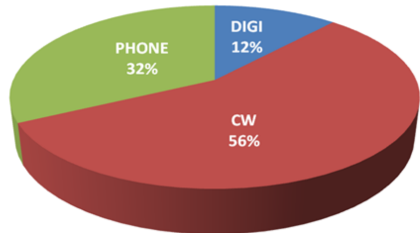
FD 2015: Score Per Mode(%)
